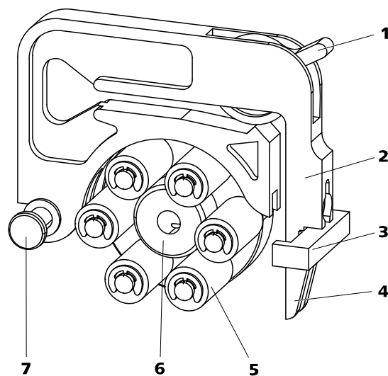
图 15 蠕动泵
